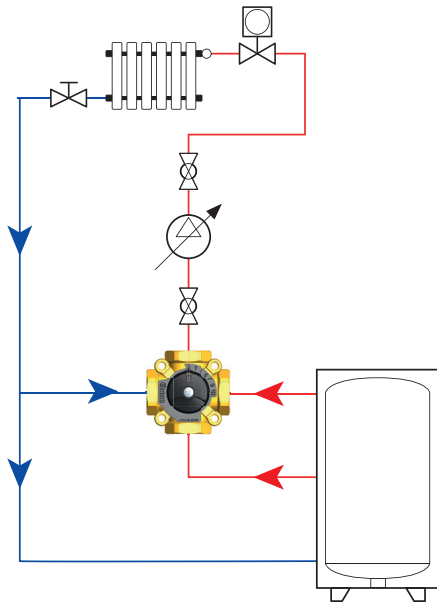
Einsatz von V52 und V53 als Mischventile
