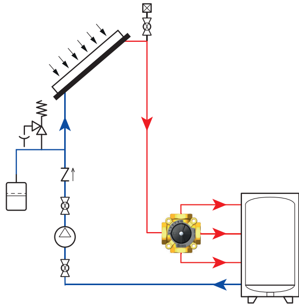
Einsatz von V52 und V53 als Umleitventile
